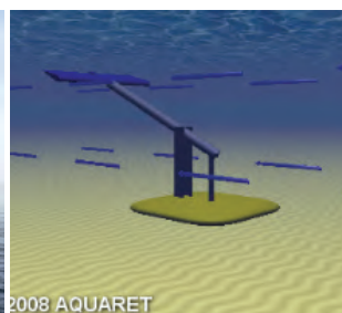
Hydrofoil oscillant ; prototype à Bordeaux.
