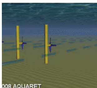
Hydrolienne à flux axial ; prototype sur l'île d'Ouessant.
